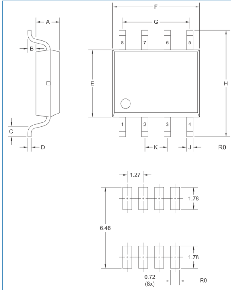
图 7-1 SOP8 封装尺寸图
