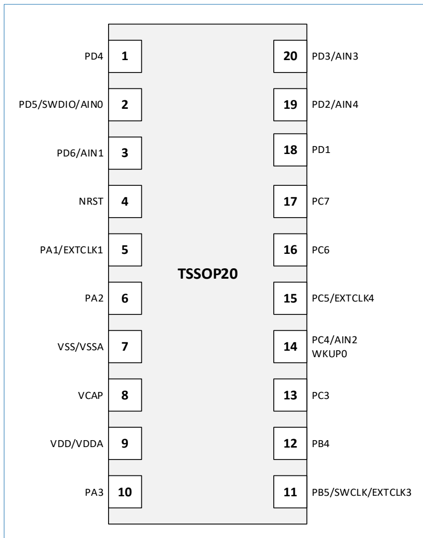
图 6-3 TSSOP20 封装
