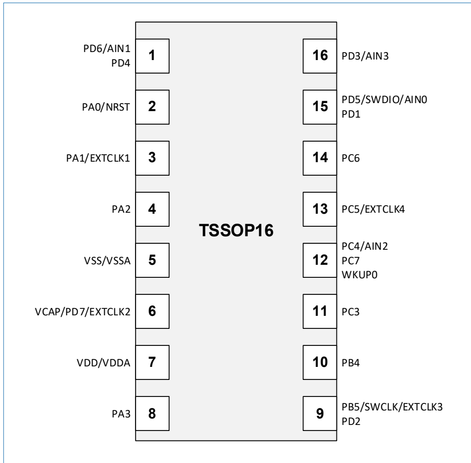
图 6-2 TSSOP16 封装
