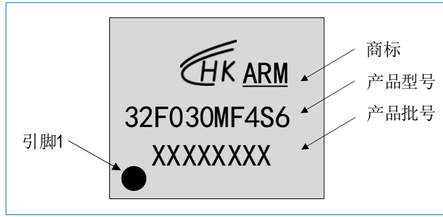
图 7-12 QFN20 HK32F030MF4S6 丝印示例
