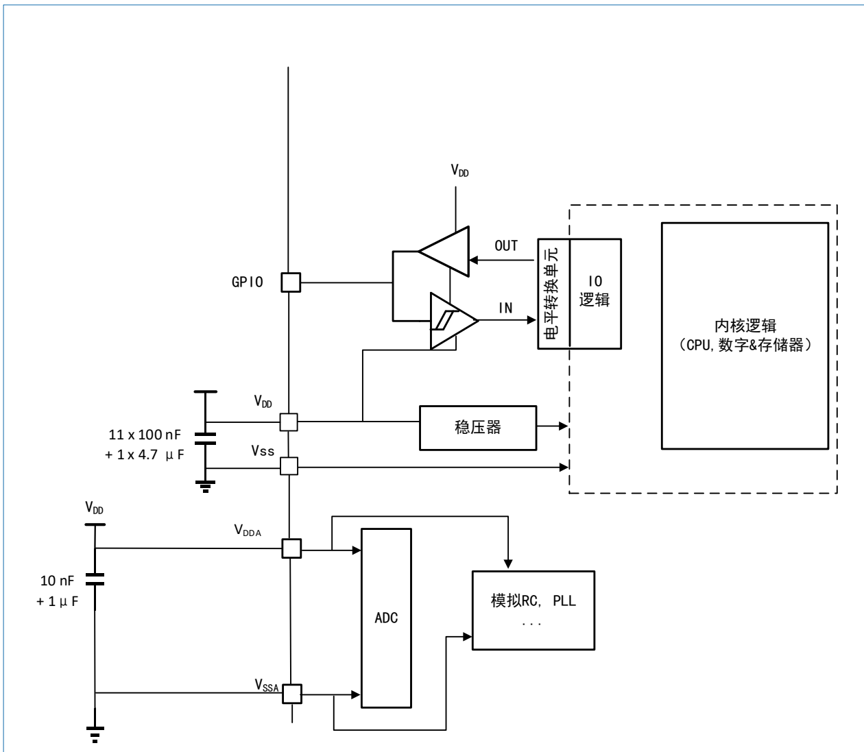
图 5-1 电源供电参考电路
