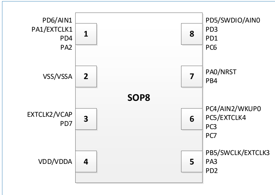
图 6-1 SOP8 封装
