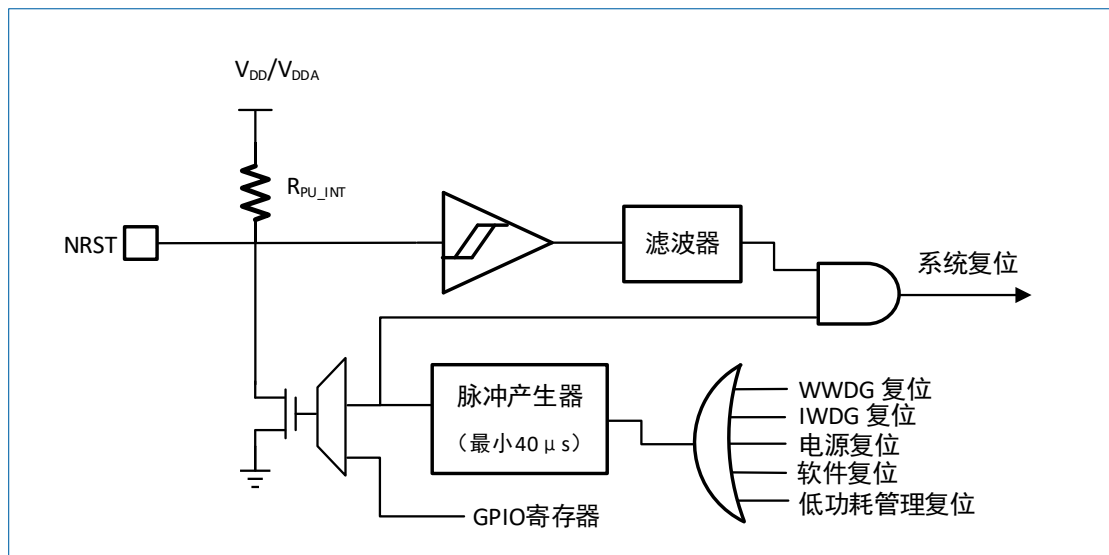
图 3-3 复位电路
