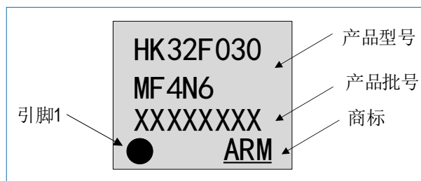
图 7-10 QFN20 HK32F030MF4N6 丝印示例
