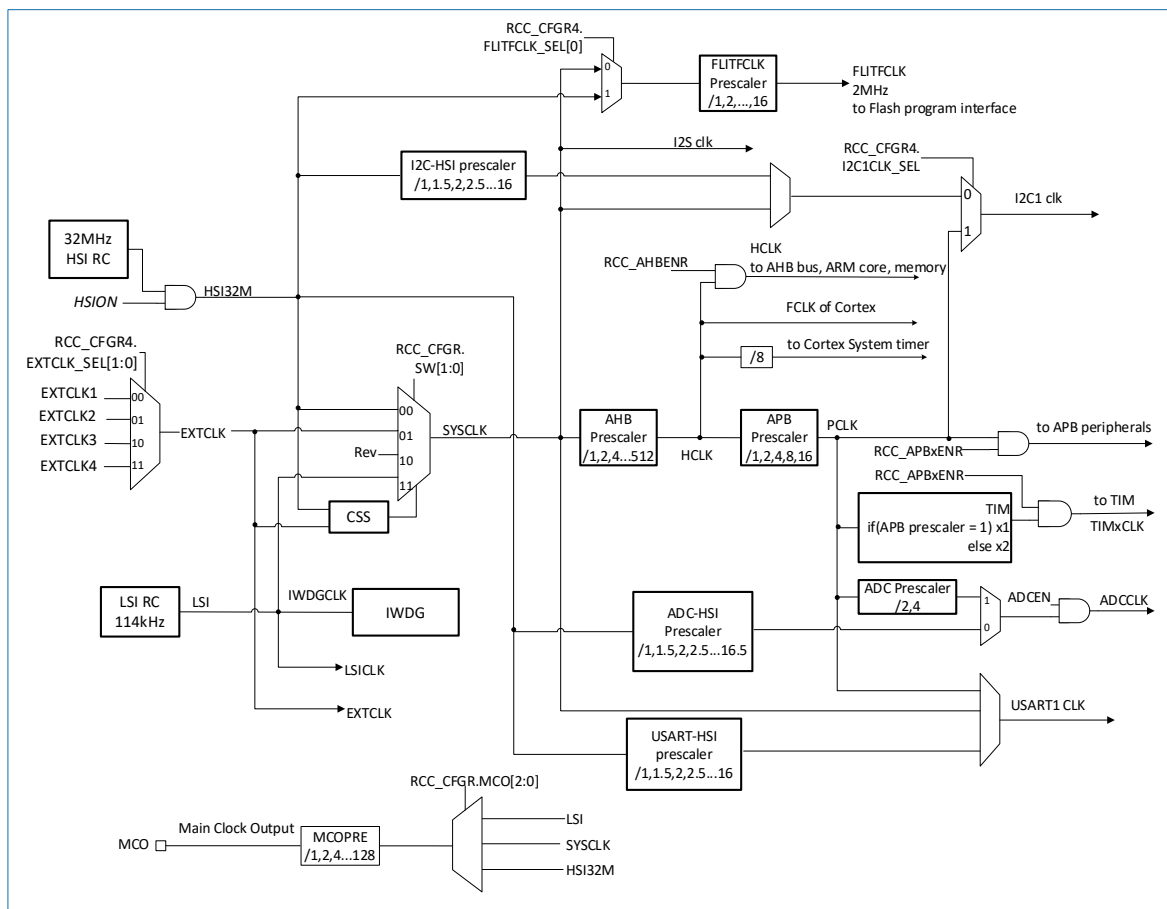
图 3-4 时钟树
