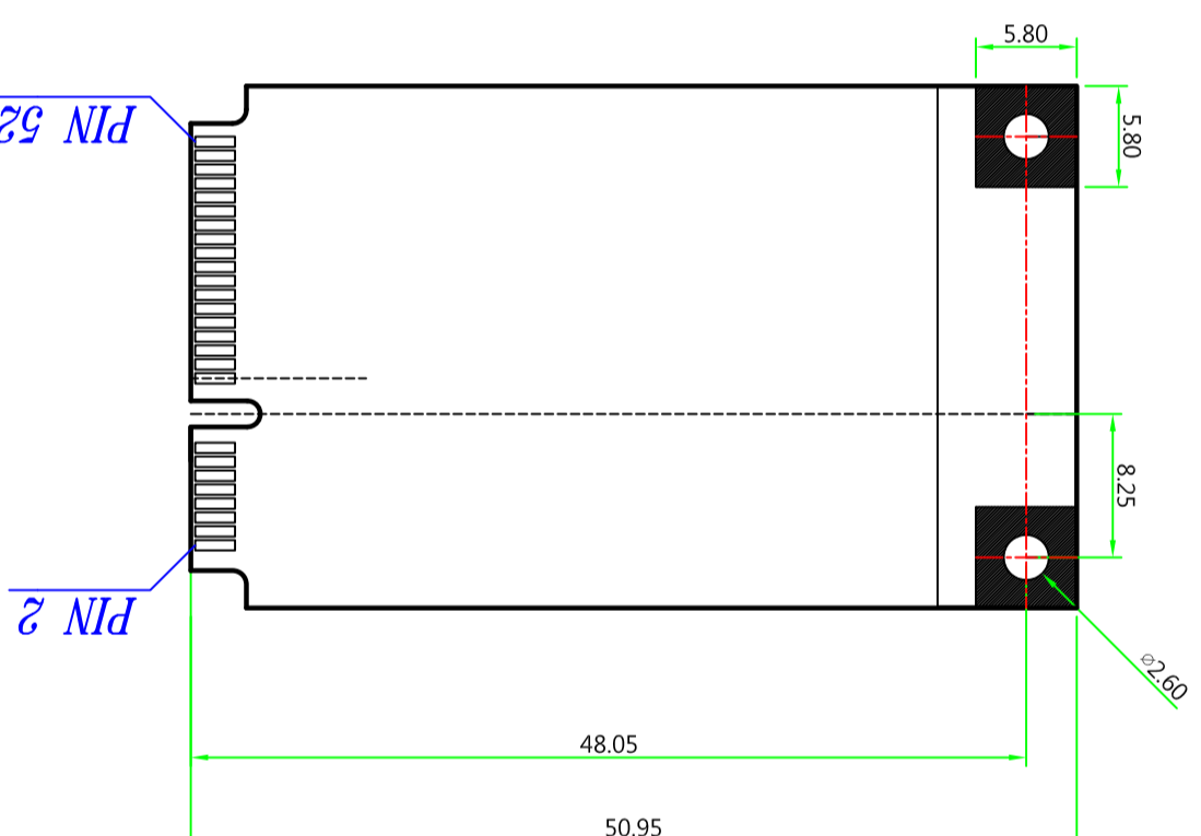
Mini PCI-E Card Bottom Side 背面
