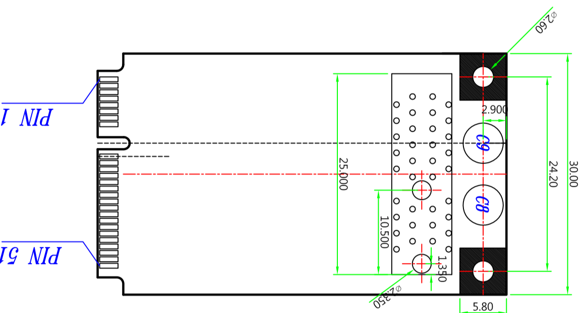
Mini PCI-E Card Top Side 正面
